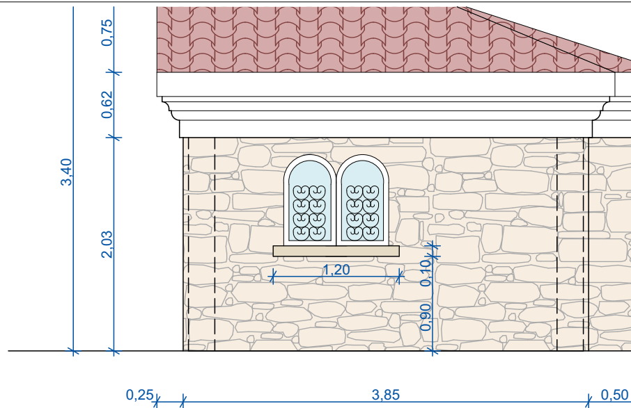
Фасада Север
