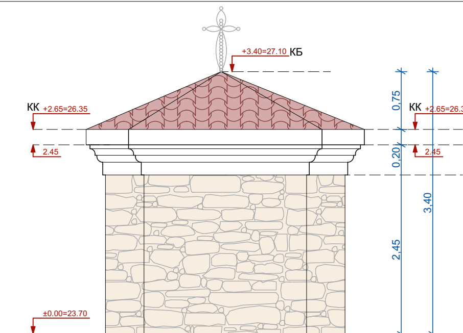
Фасада Изток
