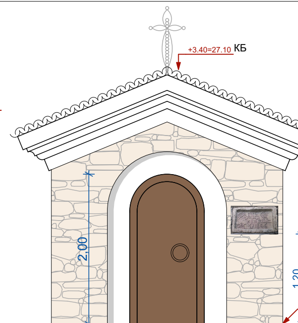
Фасада Запад
