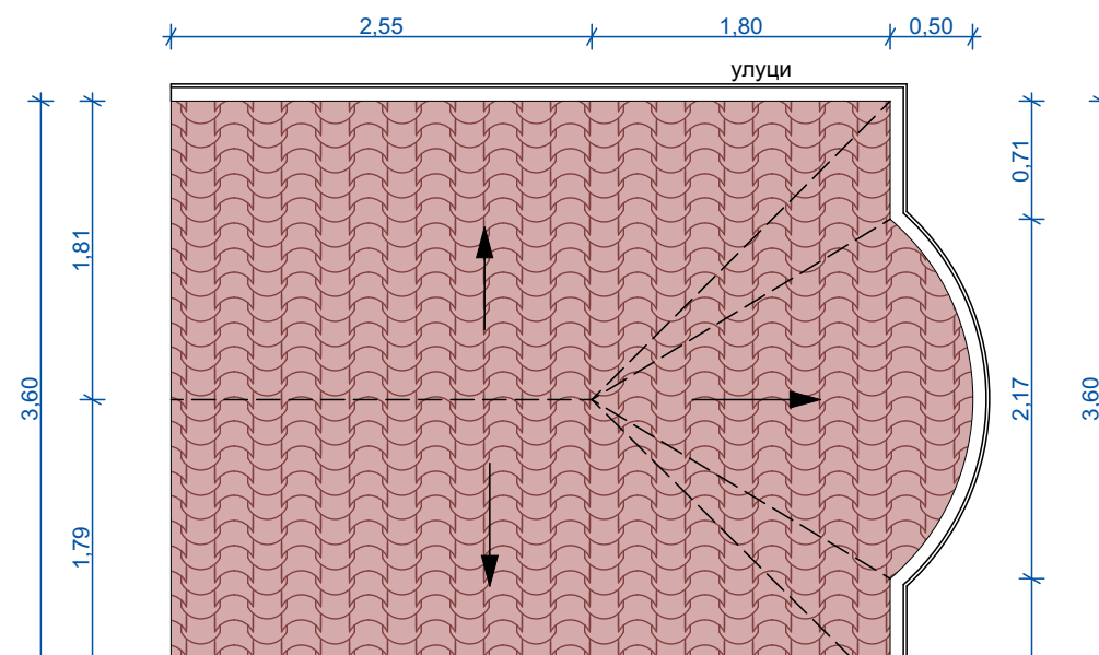
Покрив
